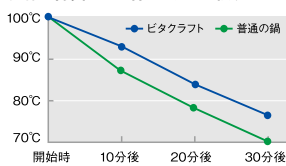
◎ 鍋の材質による保温力の比較(自社調べ)
