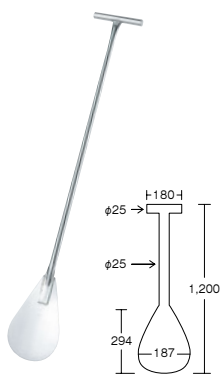
② EBM 18-8 共柄 ヘラ型 給食用 シャモジ 8202400 ¥13,000 重量:1.3kg
