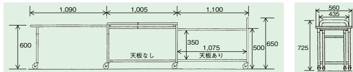
⑱18-8 給食配膳台 3連 ㊦ ㊧ ㊨ ㊩
