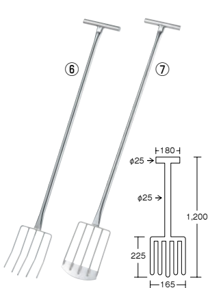
⑥ EBM 18-8 共柄 給食用 熊手フォーク 8203100 ¥12,600 重量:1.2kg
