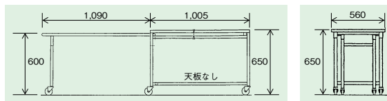
⑰18-8 給食配膳台 2連 ㊦ ㊧ ㊨ ㊩
