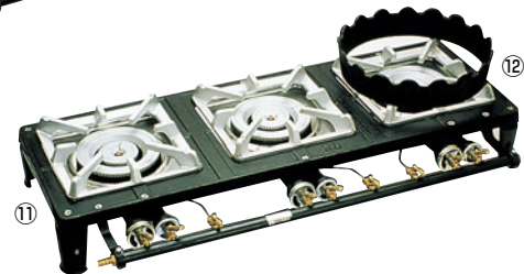
⑪ガステーブルコンロ MD-703 (3連) 直 直 ※中華用上置は、別売です。
