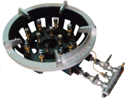
②ガスコンロ TG型 (種火付) ●パイロット(種火付) ※ご注文の際は、平型と立型のコクがございましたらご指定ください。
